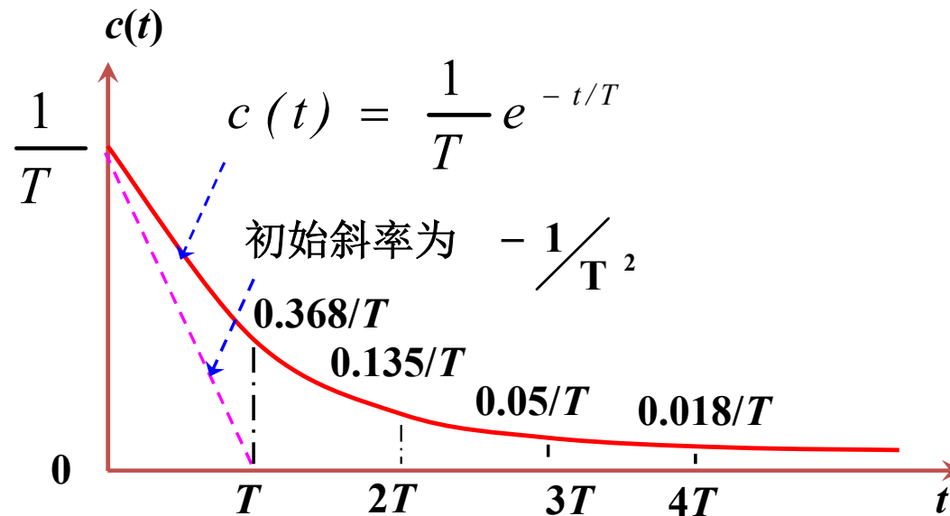
单位脉冲响应曲线
